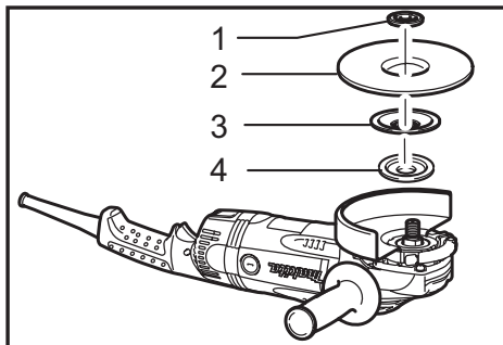
► 1. Contratuercia 2. Disco flexible 3. Plato de goma 4. Brida interior
